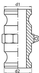
Dvojitá vsuvka (spojka) CAMLOCK
