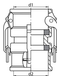
Dvojitá spojka (spojka) CAMLOCK
