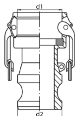
Redukce spojka-vsuvka CAMLOCK
