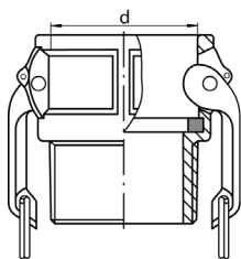
Spojka CAMLOCK s vnějším závětem BSPT nebo NPT
