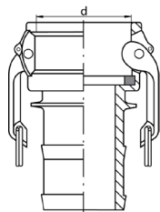
Spojka CAMLOCK s ozubeným hadicovým trnem
