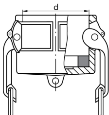
Zaslepovací víčko vsuvky CAMLOCK
