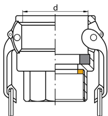
Spojka CAMLOCK s vnitřním Závitem BSP ISO-228-1
