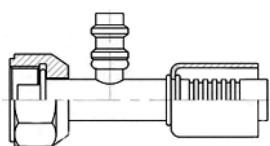
Koncovka s vnitřním závitem UNF, trubková, s ventilem R134 nízkotlakým (LP) a vysokotlakým (HP)
