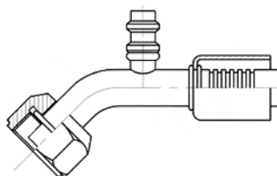
Koncovka s vnitřním závitem UNF, trubková, s ventilem R134 nízkotlakým (LP) a vysokotlakým (HP)
