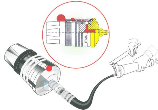
Mazací vsuvky
