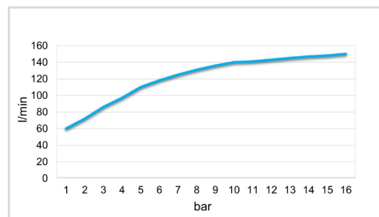
Průtok v závislosti na tlaku při plně otevřené trysce
