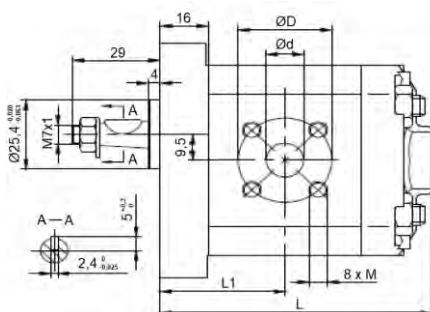
Skupina 1 - kužel 1:8, deska evropská (Ø 25,4 mm), přírubové přípojky
