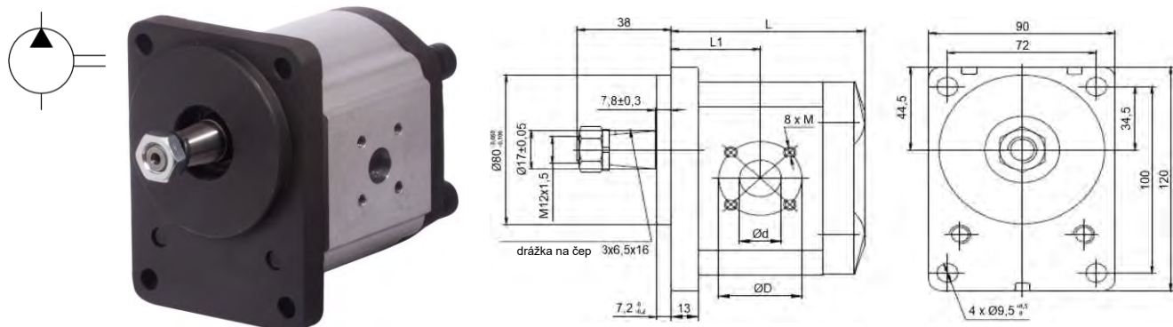
Skupina 2 - kužel 1:5, deska německá (Ø 80 mm), přírubové připojky
