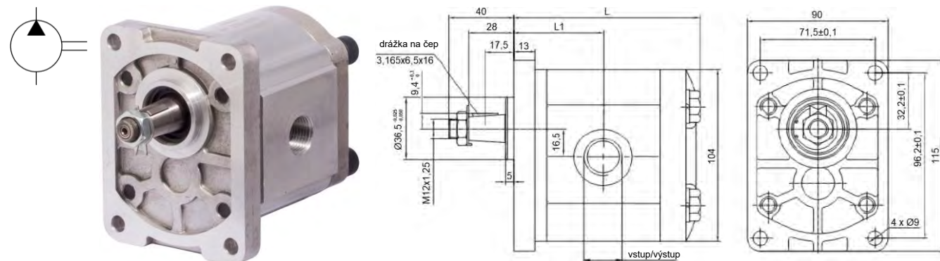
Skupina 2 - kužel 1:8, deska evropská (Ø 36,5 mm), závitové připojky
