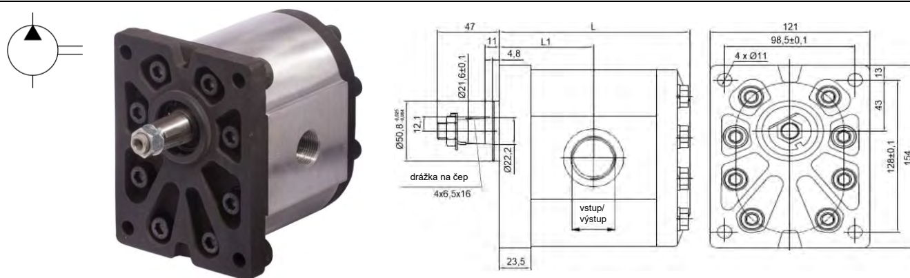
Skupina 3 - kužel 1:8, deska evropská (Ø 50,8 mm), závitové přípojky
