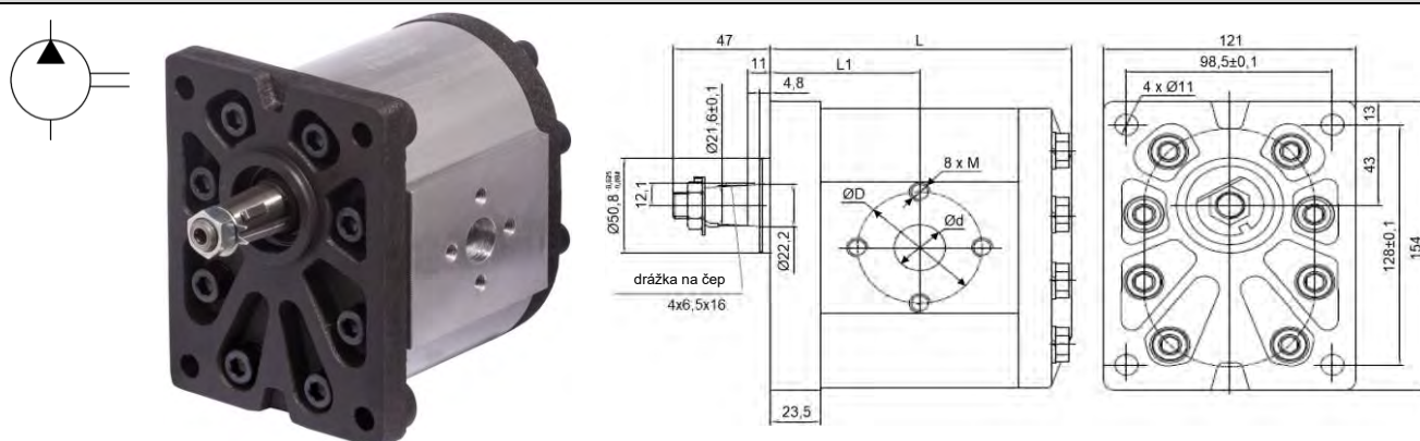
Skupina 3 - kužel 1:8, deska evropská (Ø 50,8 mm), přírubové přípojky
