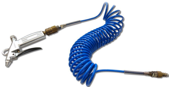
Sada – hliníková vzduchová pistole s regulací průtoku napojená na spirálovou hadici pomocí rychlospojek Eurostandard DN7,2
